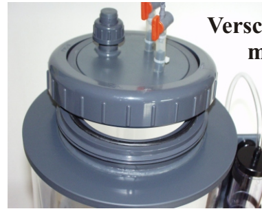
Sonden- einschub PH Entlüftung Entnahme
